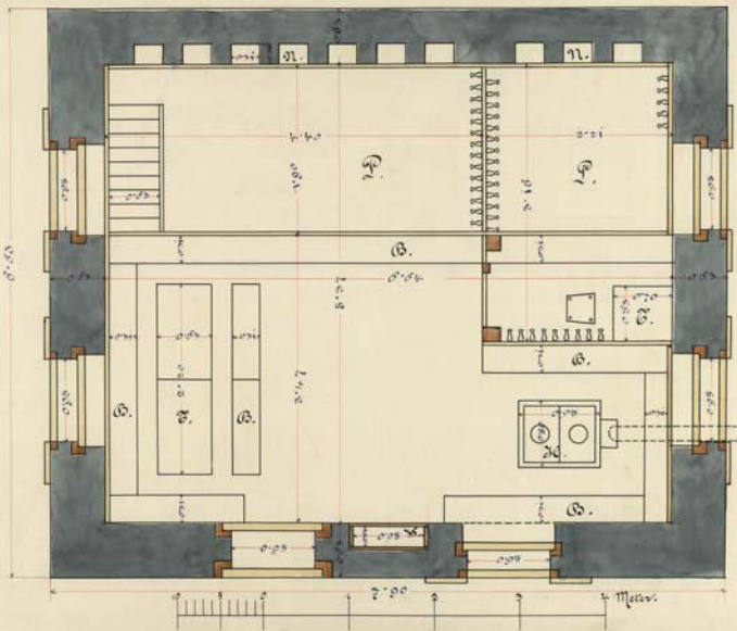
Grund- und Aufrissplan des ersten Baus der Alten Prager Hütte von 1872
