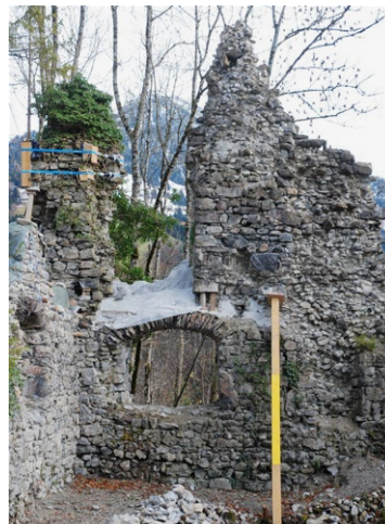
Palas Nordostecke innen, Sicherungen
